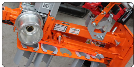
Carry-Rack for Conduit adaptors
